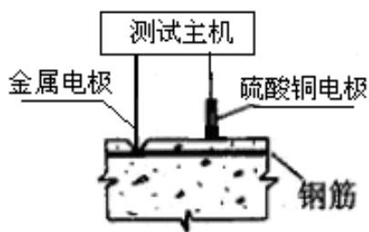
图 5-4 钢筋锈蚀仪电位测量方式示意图
