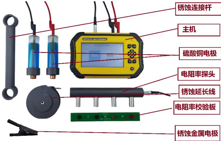
图 1-1 仪器的组成
